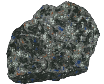
gabro
