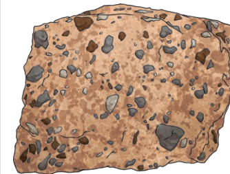
brecha
