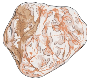
mármol
