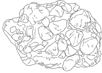
conglomerado
