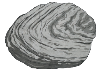
gneis
