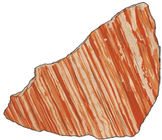
arenisca
